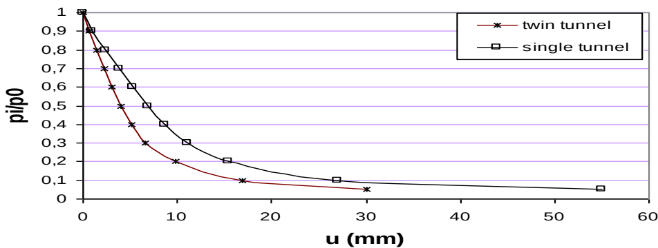
شکل ۶: منحنی مشخصه زمین (GRC) برای توده سنگ در وضعیت (۳)
