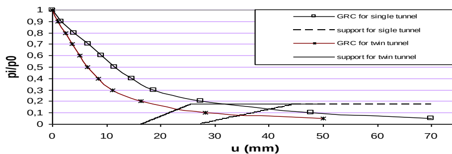
شکل ۹: منحنی اندرکنش زمین و سیستم نگهدارنده در وضعیت (۱)
