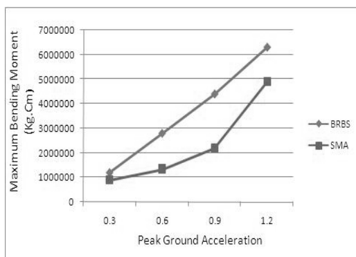
شکل ۲۹- نمودار حداکثر لنگر خمشی ستون‌های طبقه اول بر حسب حداکثر شتاب زمین
