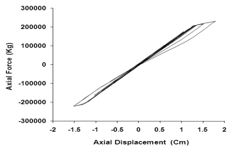
شکل ۷- نمودار نیرو- تغییر مکان محوری بادبندهای طبقه اول در سیستم SMA تحت حداکثر شتاب افقی 0.6g
