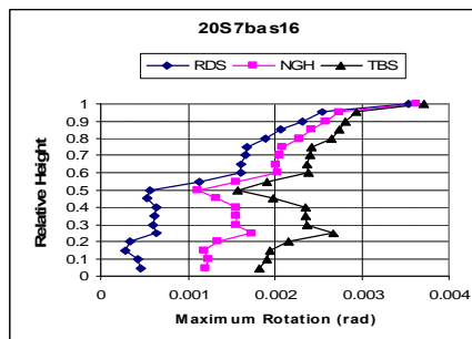
ق- بررسی در قاب ۲۰ طبقه با مهاربندی X در ۴ طبقه
