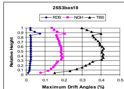
ق- بررسی در قاب ۲۵ طبقه با مهاربندی X در ۷ طبقه
