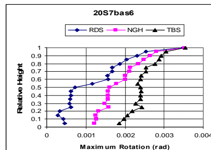
ح- بررسی در قاب ۲۰ طبقه با مهاربندی X در ۱۴ طبقه
