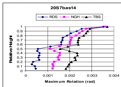
ف- بررسی در قاب ۲۰ طبقه با مهاربندی X در ۶ طبقه
