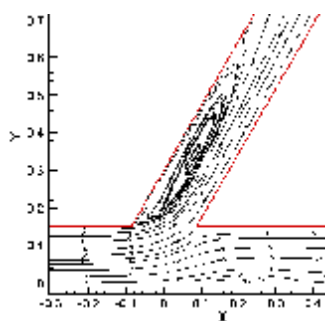
شکل ۱۷: خطوط جریان در R=0.52 و \theta=60 .
