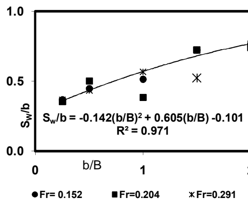
شکل ۱۱: رابطه بین S_W/b و b/B در R=0.31 .
