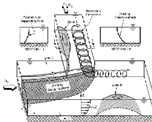
شکل ۱: الگوی سه بعدی جریان در آنگیرهای جانبی [۱].
