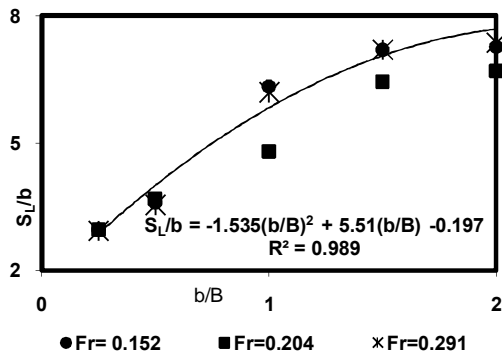
شکل ۱۲: رابطه بین S_L/b و b/B در R=0.31 .
