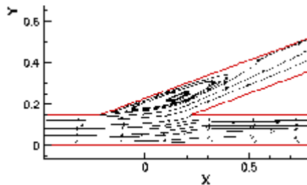
شکل ۱۳: خطوط جریان در R=0.31 و \theta=30 .
