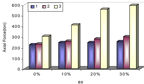
شکل ۲: نیروی محوری فشاری ستون شماره ۱ در سازه دارای جداگر تیب ۱ تحت زلزله بم.
