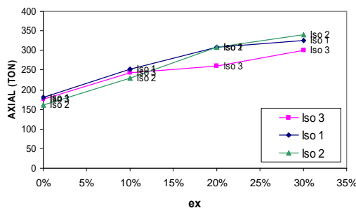
شکل ۴: مقایسه نیروی محوری فشاری ستون شماره ۱ در سه تیب جداگر تحت زلزله السنترو.
