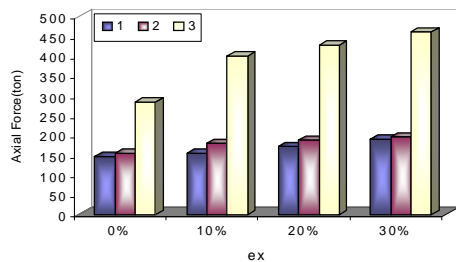
شکل ۳: نیروی محوری فشاری ستون شماره ۱ در سازه دارای جداگر تیب ۳ تحت زلزله بم.
