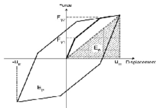
شکل ۲۲: الگوی مناسب محاسبه میرایی معادل اتصالات [۱۲].
