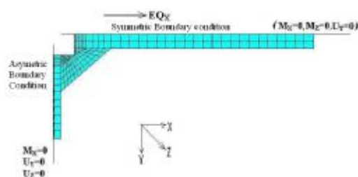
شکل ۳: مدل نمایشگر \frac{1}{4} اتصال با ورق مثلی در پلان.
