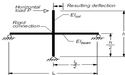
شکل ۱: مدل پیشنهادی آزمایشگاهی اتصال مطابق مرجع [۱].
