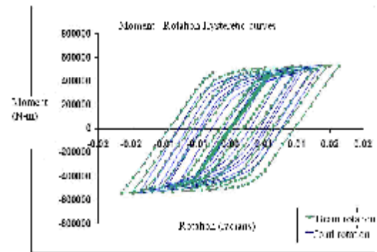
شکل ۲۰: مدل نهم- اتصال تیر شامل منطقه تضعیف‌شده شبه استخوانی به ستون دارای ورق پیوستگی داخلی.
