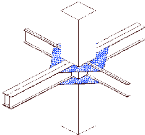
شکل ۴: نمایش شماتیک ورق‌های تقویتی مثلثی پیرامونی ستون قوطی شکل (مدل شماره ۳).
